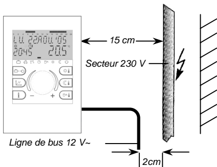
Schéma 1 : Ecarts minimum pour installation électrique
