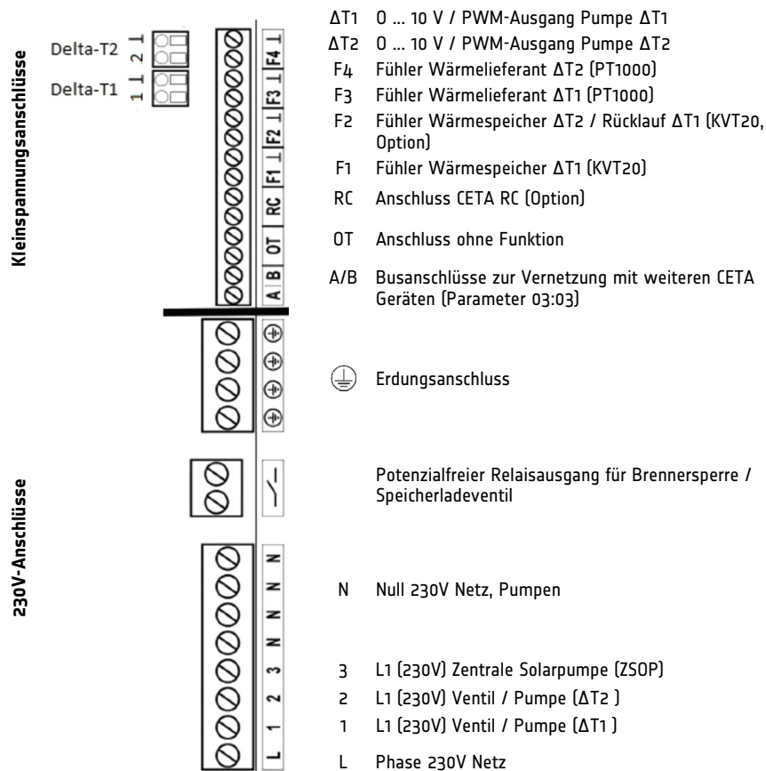
Abb. 8: Elektrische Anschlüsse
