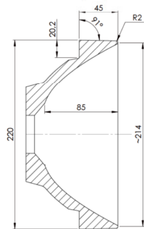
B-B (1 : 2)
